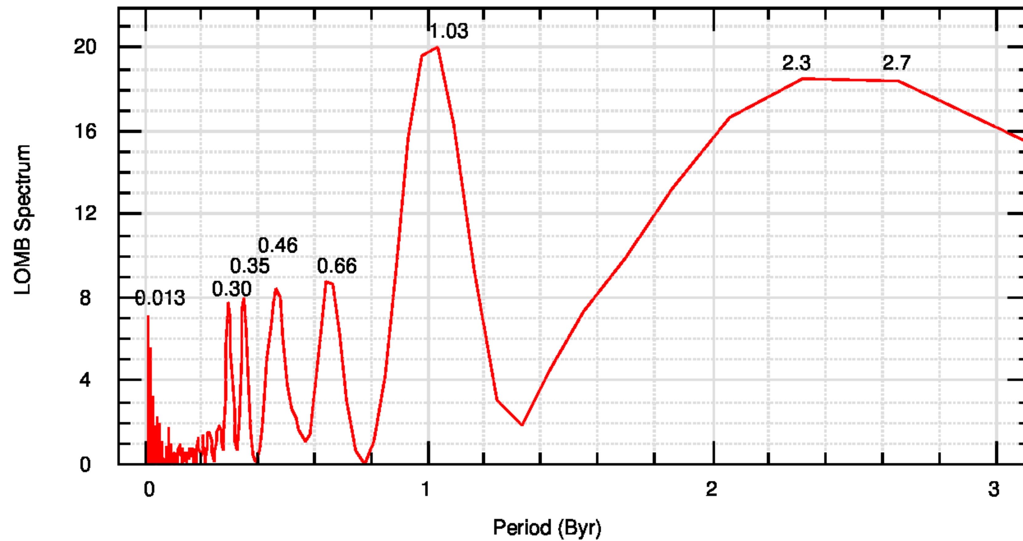
d13C-21
