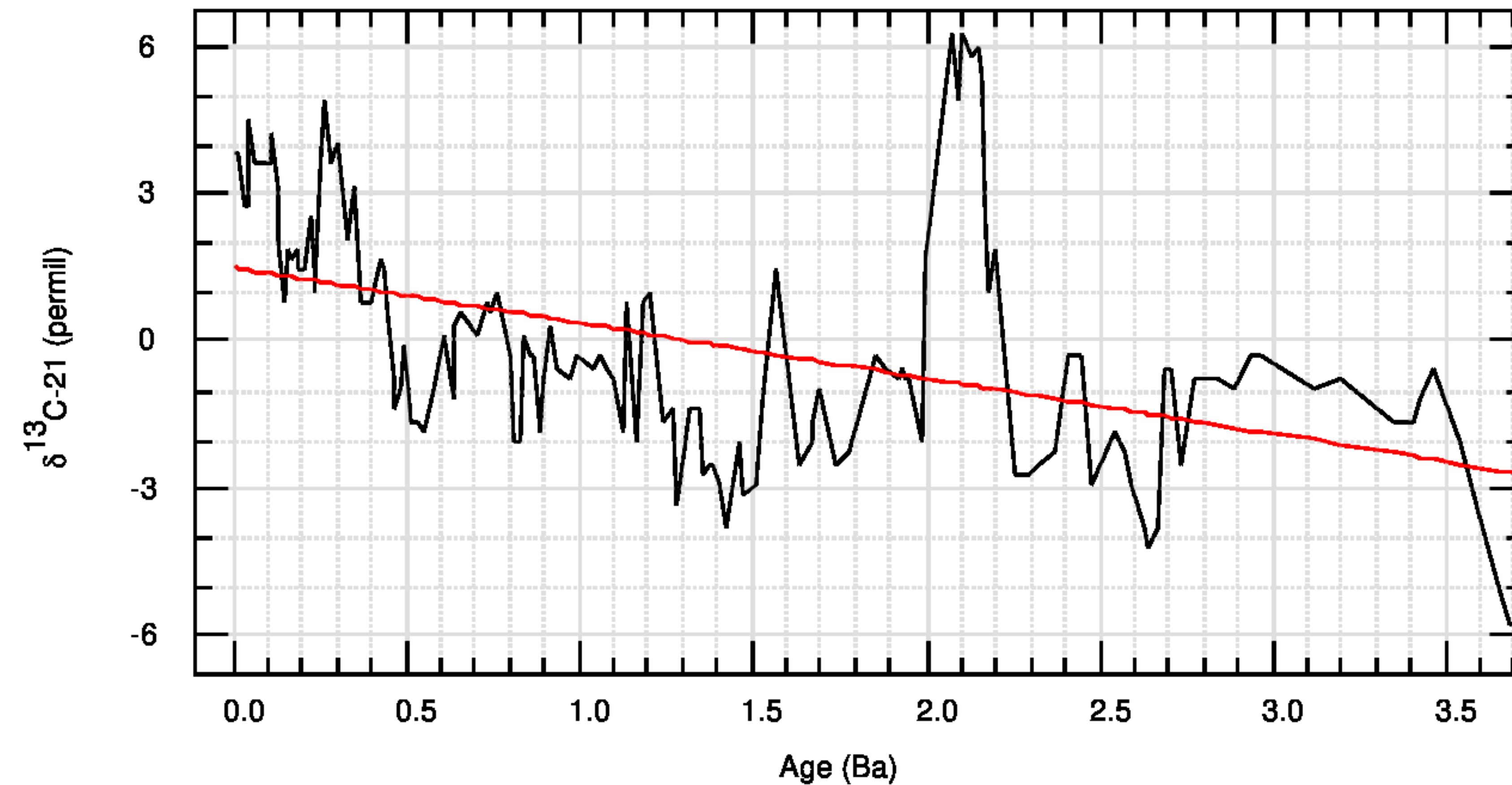
d13C-21
