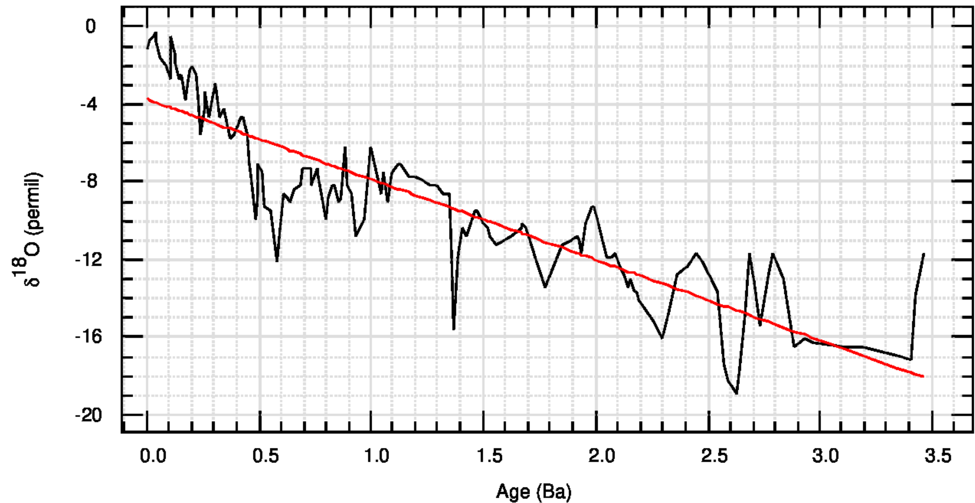
d18O-21
