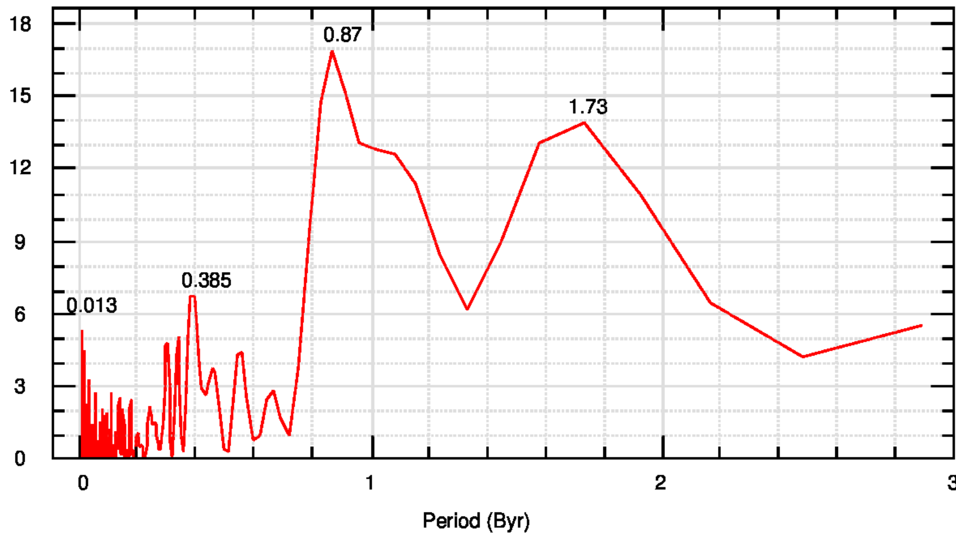
d18O-21
